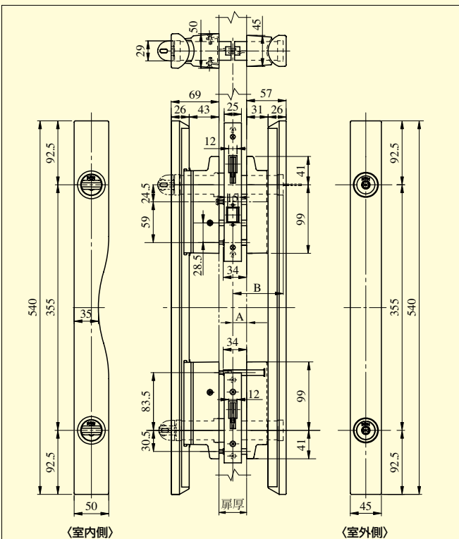
【外形図】
